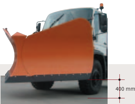
Baureihe V im angehobenen Zustand
