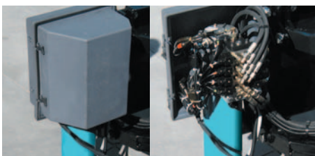
Elektro-hydraulische Steuerung
